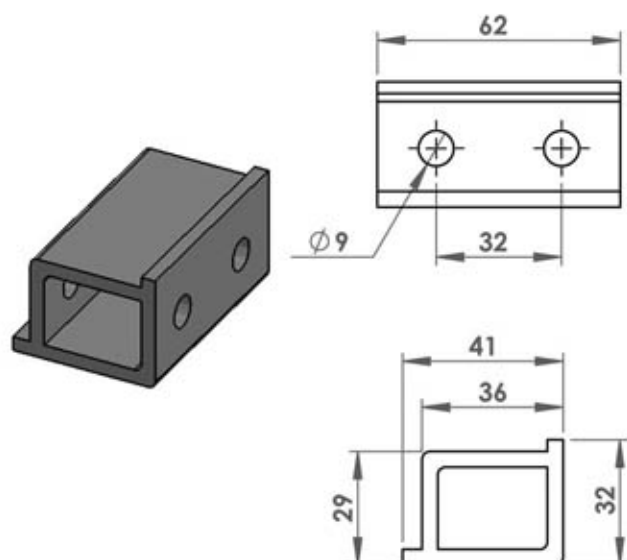
500 10 500 Gâche latérale brute à souder Side raw steel keeper to be welded
