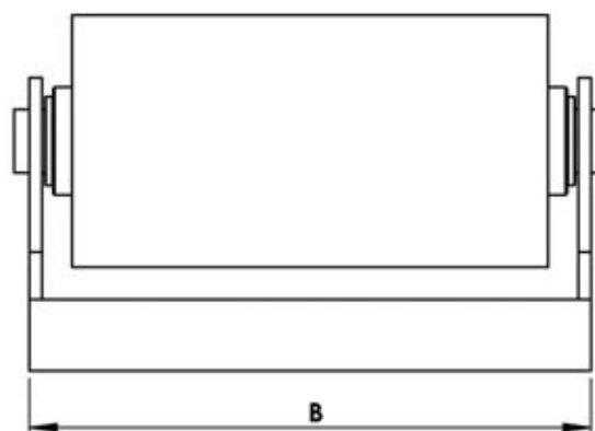
Montage avec bagues ERTALON Assembled with ERTALON
