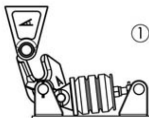
Fig. n°1: Position de l'AFHYX lorsque l'axe de verrouillage de la benne vient en contact avec le crochet.
